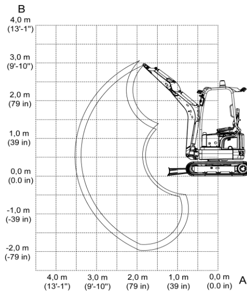
Abb. 1: Hubkrafttabelle EZ17e
